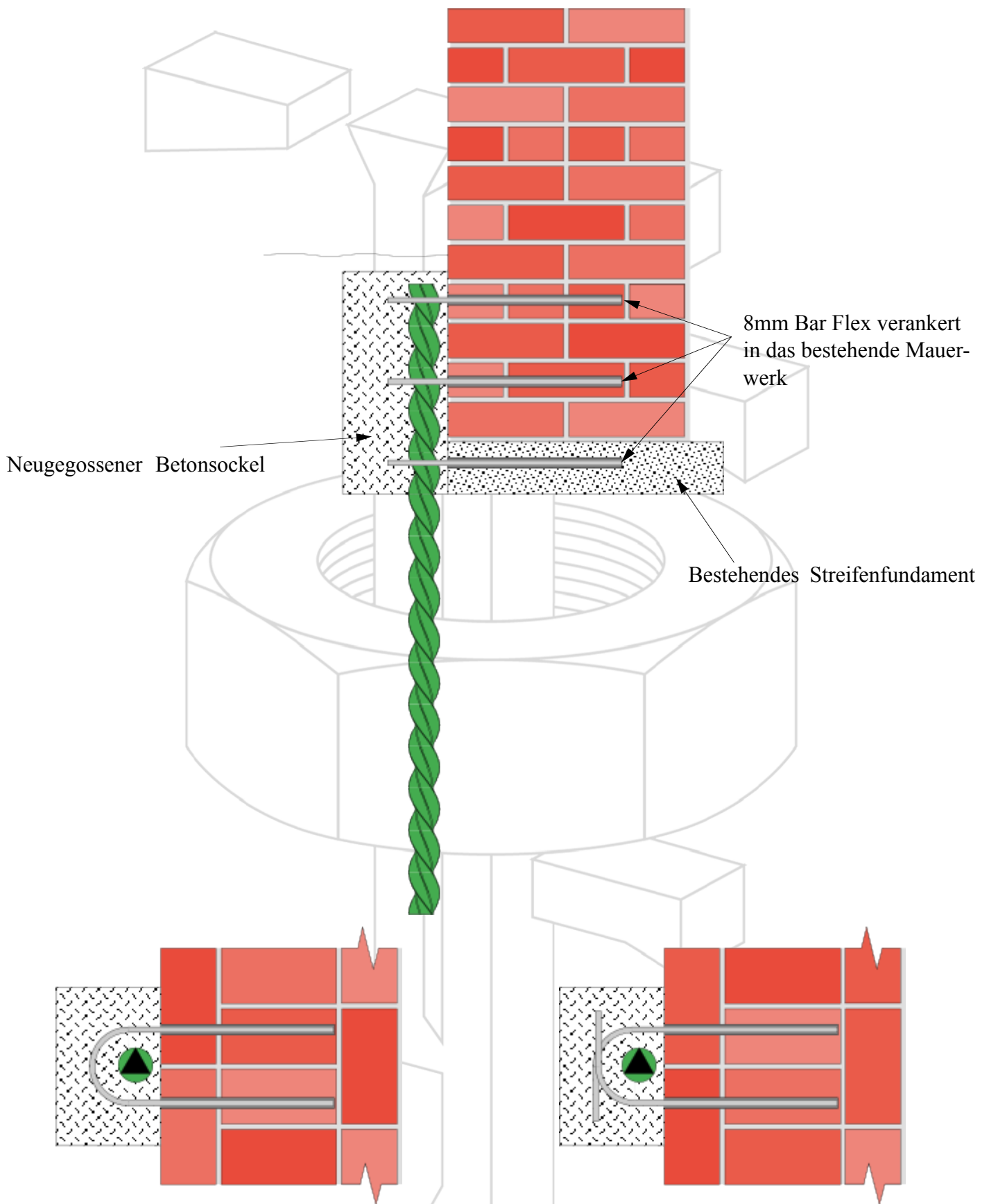
Draufsichten alternativer Methoden für die Befestigung der Verankerung
